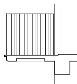
Fig. 3: Altanbund i eksempelvis beton (snit) kan udføres med udsparringer på underside og/eller profilering i forkant.
